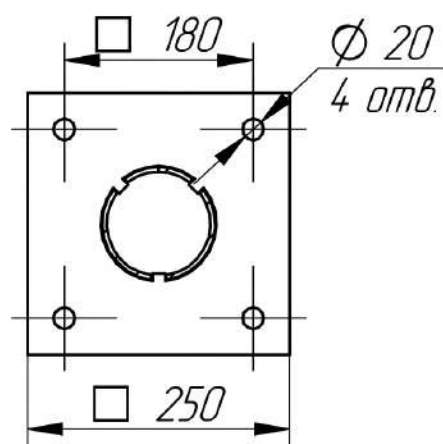
Фланец основания
